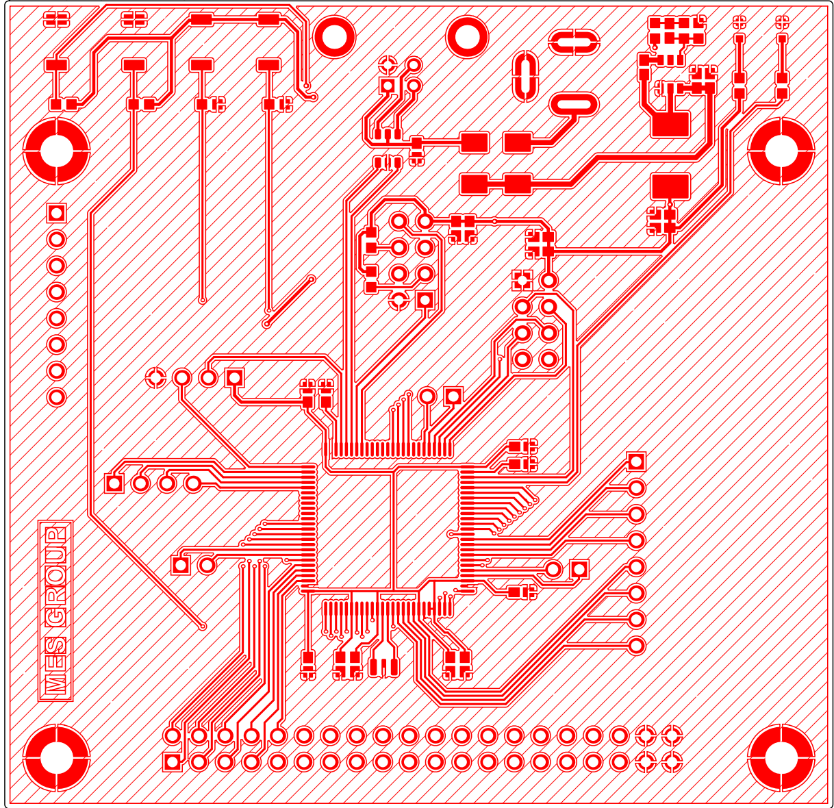
Top Layer (Scale 2:1)
