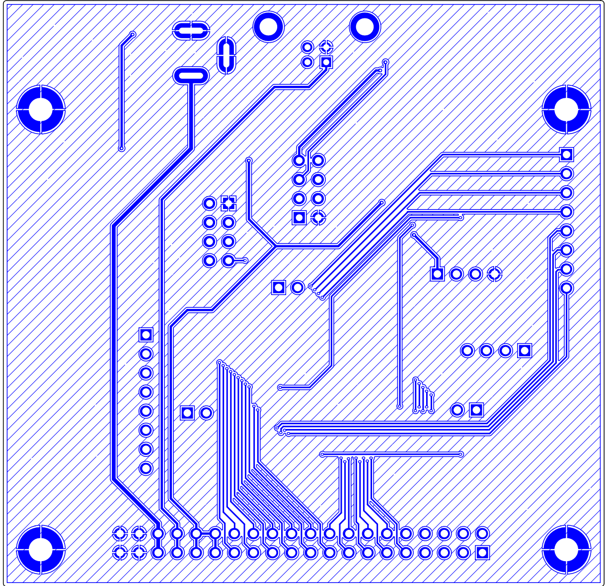
Bottom Layer (Scale 2:1)
